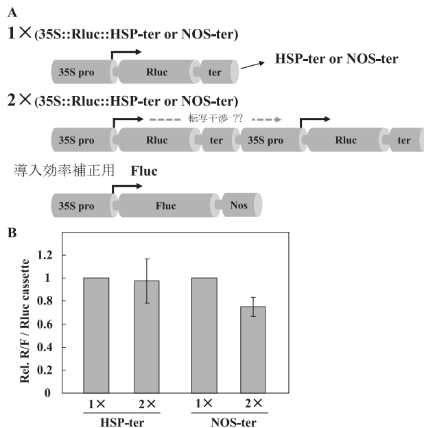
図3. ターミネーターの違いが下流遺伝子の発現量に及ぼす影響。A) 一過性発現実験に用いた構築図。B) 一つの発現カセットあたりのRluc発現量。Nos-terの場合、上流の発現カセットからの発現量が同じとすると、下流からの発現量は半分となる。
