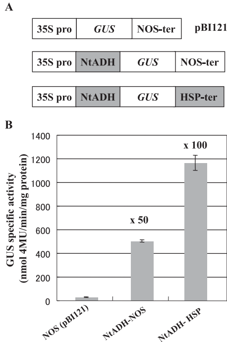
図4. 完全なシングルコピー導入個体での導入遺伝子発現量の比較. A) バイナリーベクターの構築図. B) それぞれの個体におけるGUS比活性.
